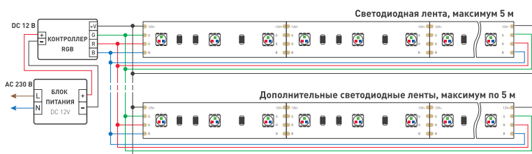
Черный провод — общий «+», красный провод — «R», зеленый провод — «G», синий провод — «B» Схема 2. Подключение нескольких светодиодных лент с двух сторон
