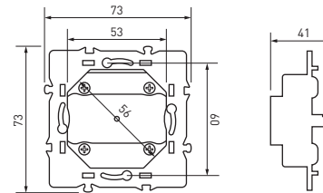
Рис. 1. Габаритный чертеж
