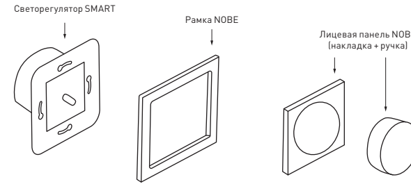
Рис. 3. Монтаж светорегулятора
