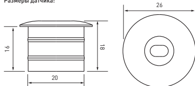
Размеры датчика:
